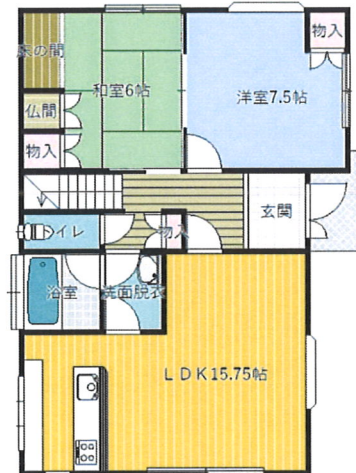
1階平面図
